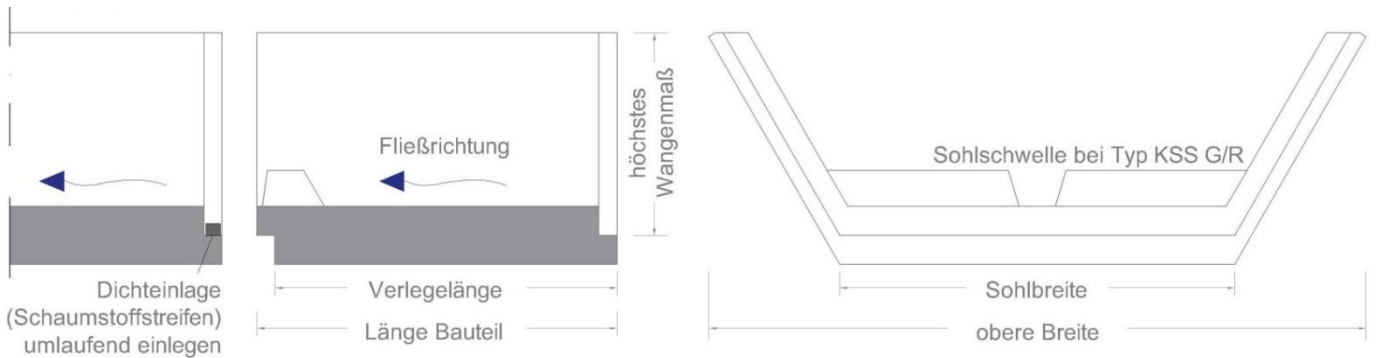
Längsschnitt
